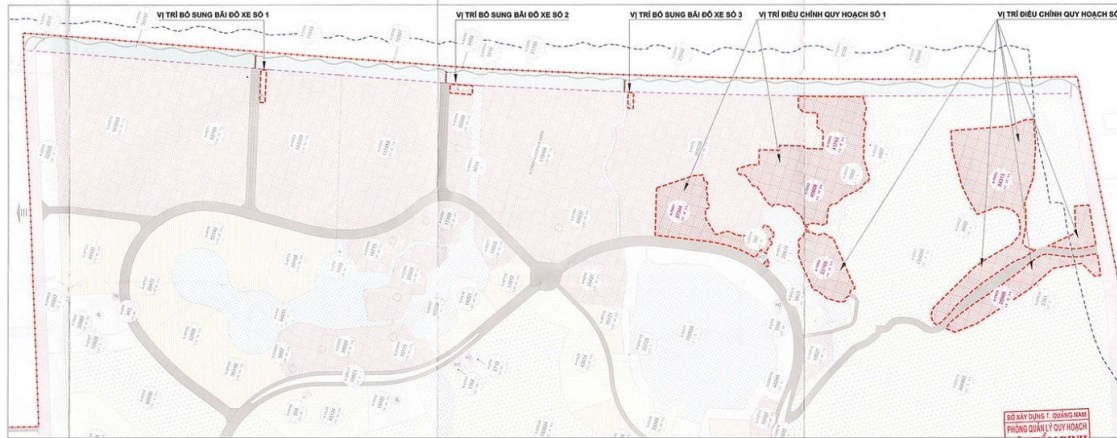
TỔNG MẶT BẰNG QUY HOẠCH SỬ DỤNG ĐẤT XIN ĐIỀU CHỈNH CỤC BỘ QUY HOẠCH PHÂN KHU (TỶ LỆ 1/2000)
